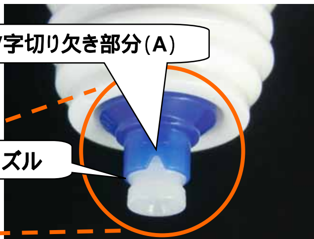
ノズル周辺の拡大写真
