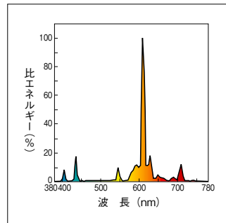
紫外線吸収膜付 (演色AAA) 白色:W-EDL・NU
