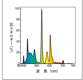
3波長形昼光色:EX-D(ED)
