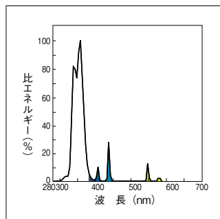
捕虫器用 (20形、40形)
