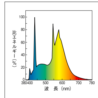
紫外線吸収膜付 (演色AA) 昼白色:N-SDL・NU
