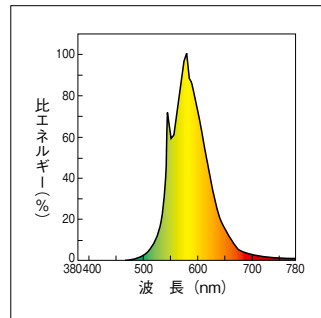
低誘虫 黄色:Y
