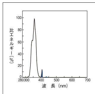
ブラックライト (FHF用)
