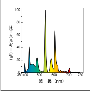
3波長形昼白色:EX-N(EN)
