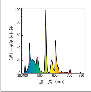
クリアデライト:EDC(3波長形昼光タイプ)
