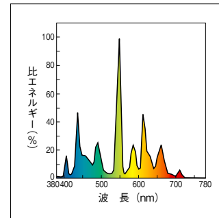
生鮮食品用 昼白色
