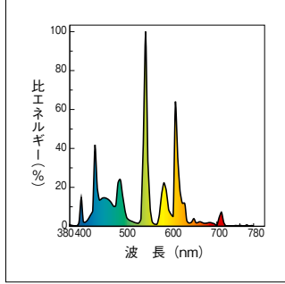
クリアナチュラルライト:ENC(3波長形昼白色)
