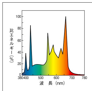
食肉展示用 温白色
