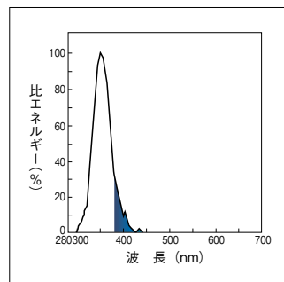
ブラックライト (FL用)
