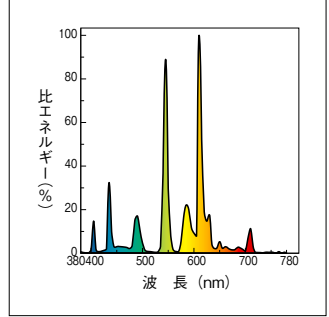
3波長形電球色:EX-L(EL)
