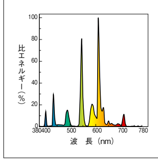
クリア電球色:ELC(3波長形電球色)
