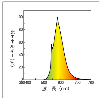
クリーンルーム用 黄色:Y
